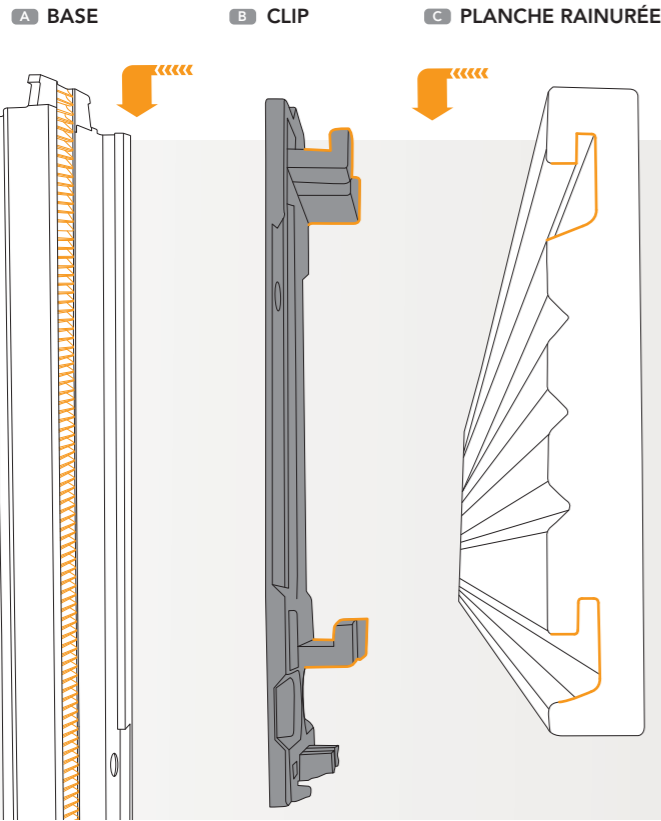
01 Fixation des bases Techniclic ®
