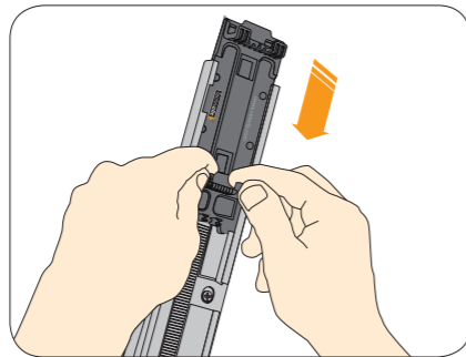
05 Pose de la lame suivante
